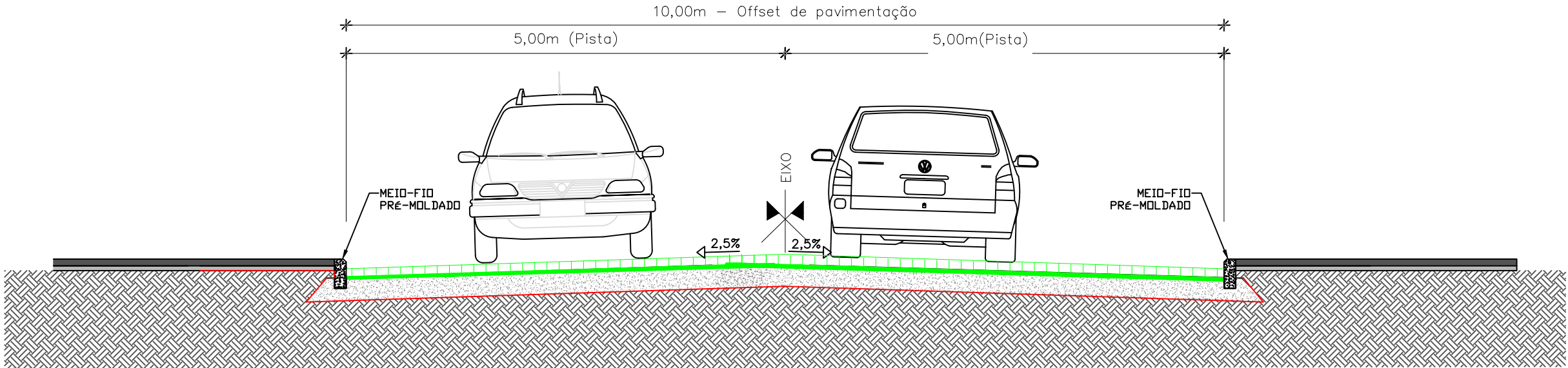
SEÇÃO TIPO DE PAVIMENTAÇÃO- Offset de pavimentação com bloco intertravado-RUA VER. OTTMAR MUENCH
